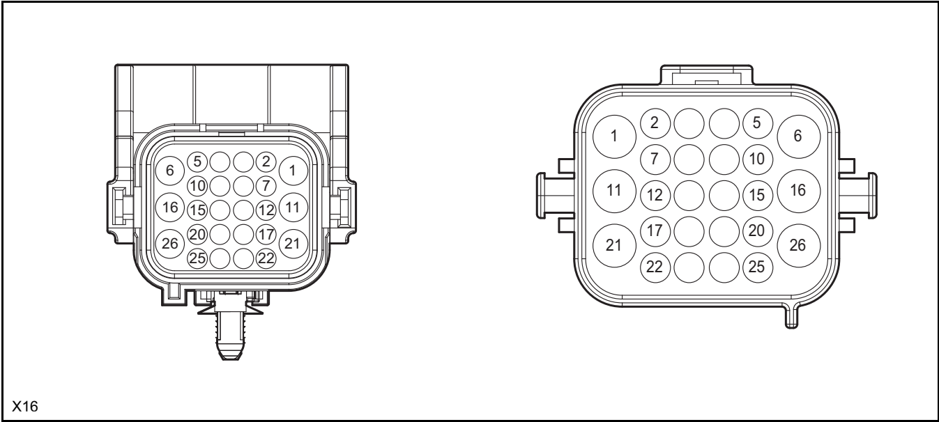
发动机舱线束接发动机线束
